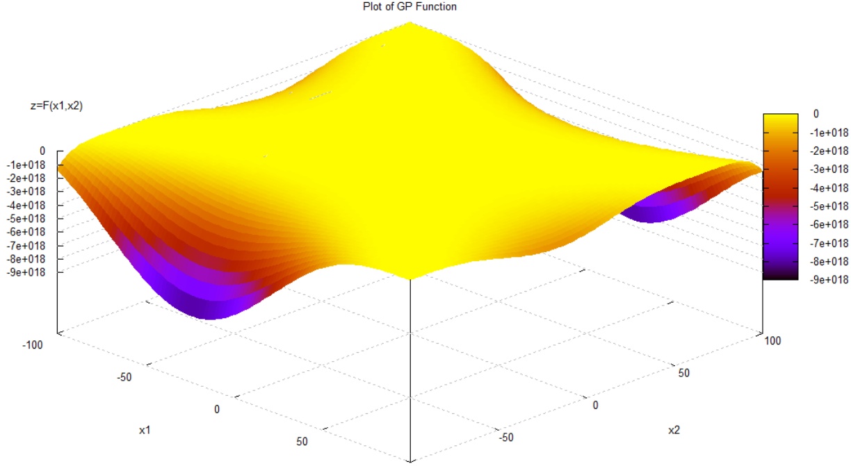
Fig. 4. Goldstein-Price (GP) Function
